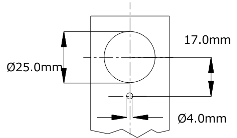
図7：取付穴の寸法
